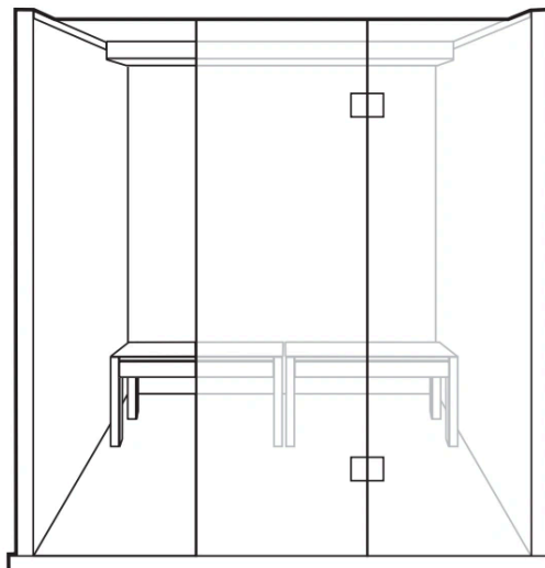
Porte et paroi avant installées
